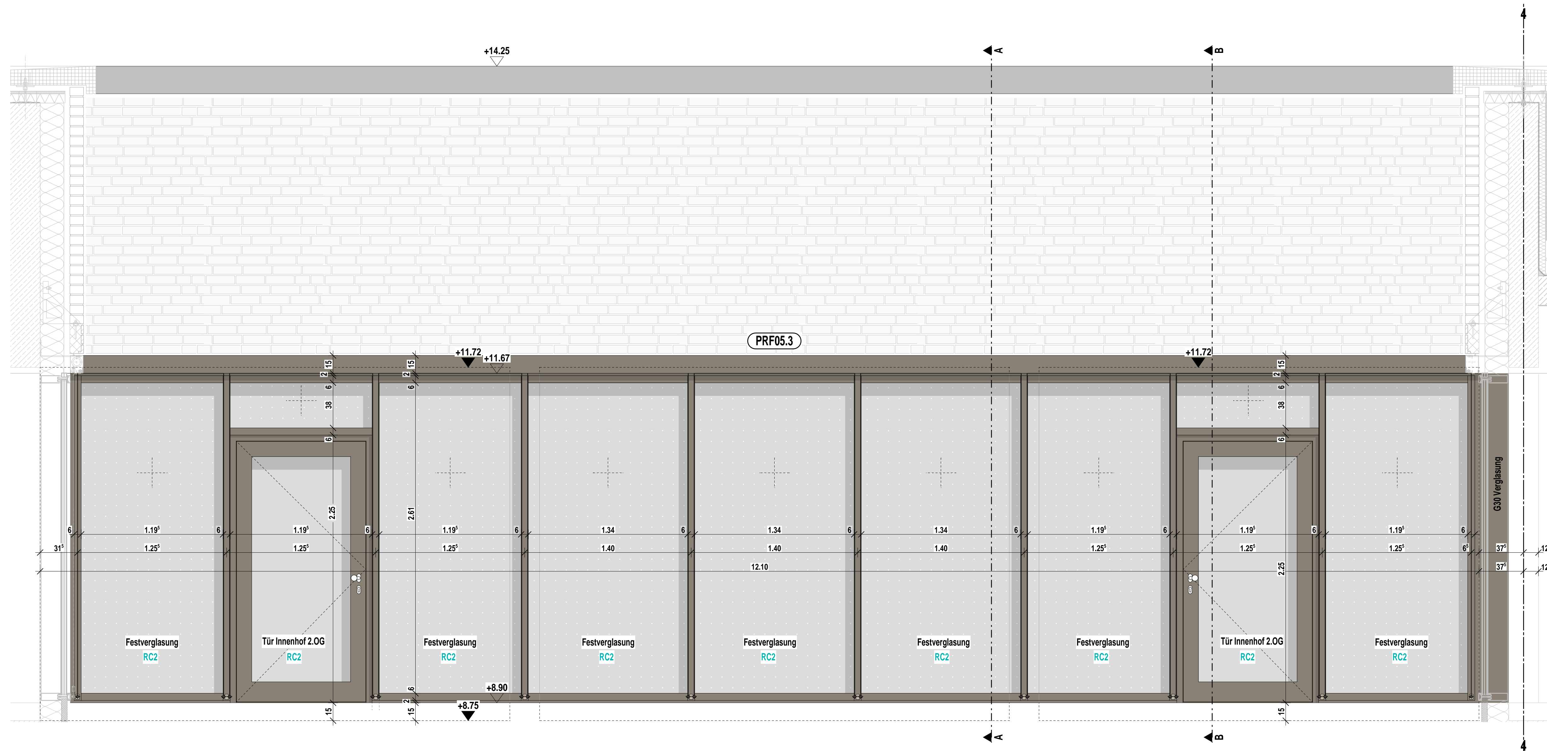
Ansicht Süd
