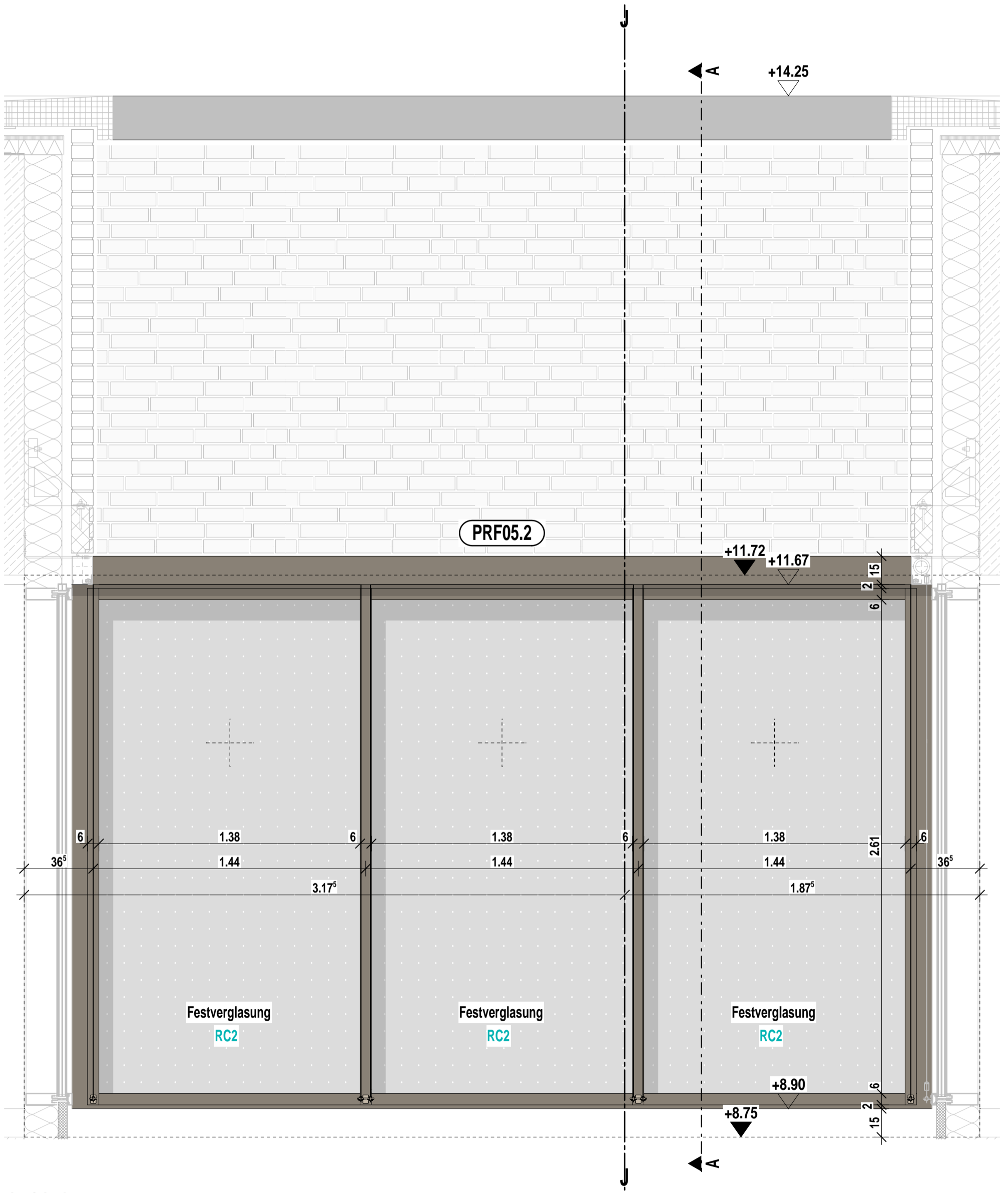
Ansicht Ost
