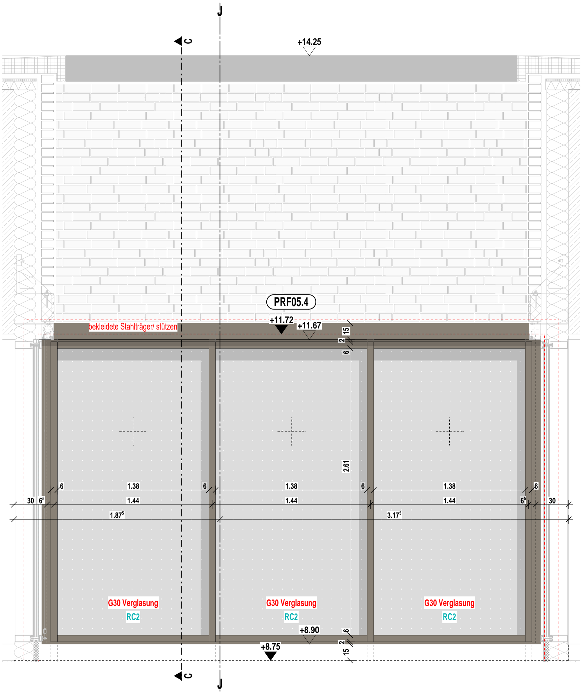
Ansicht West
